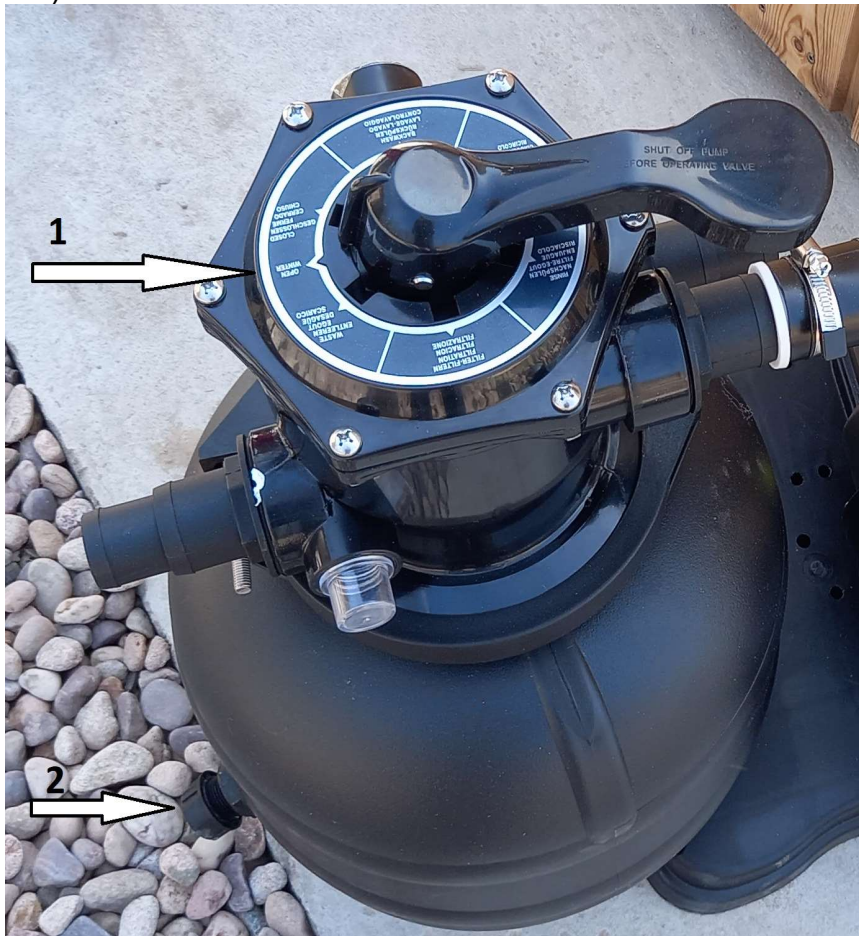
Position « OPEN WINTER » (1) et bouchon de purge du filtre (2)
